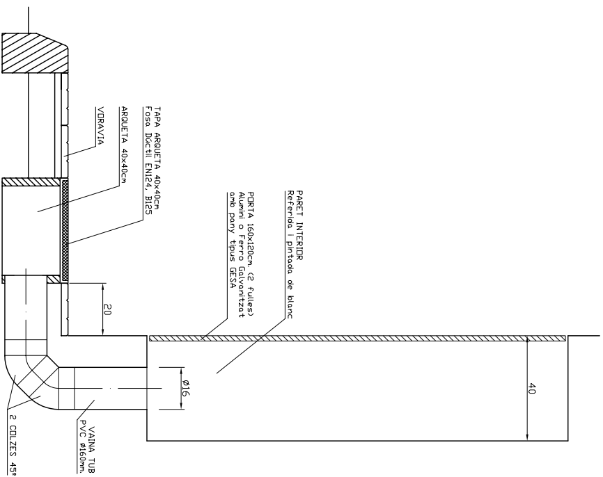
SECCIO A-B
